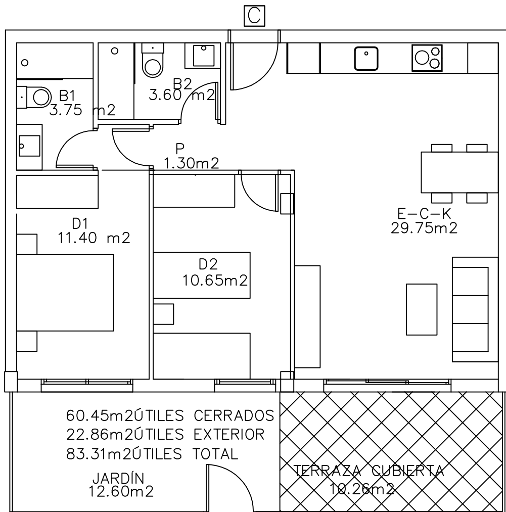
BAJO C VERSIÓN 2 DORMITORIOS
