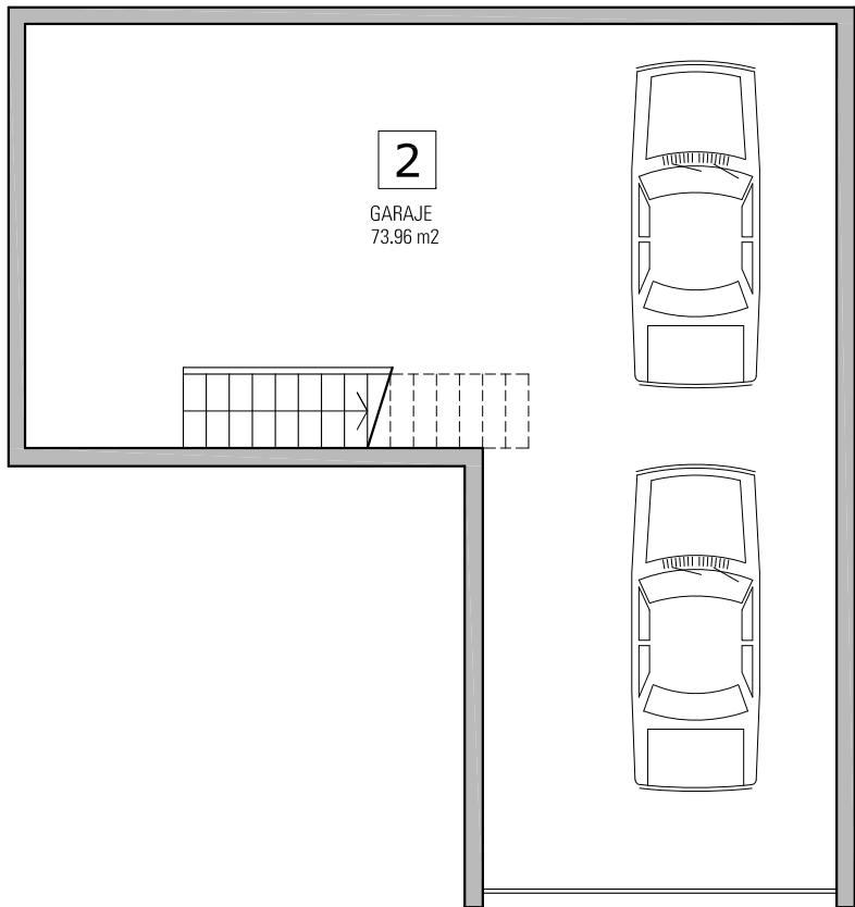
PLANTA SOTANO
