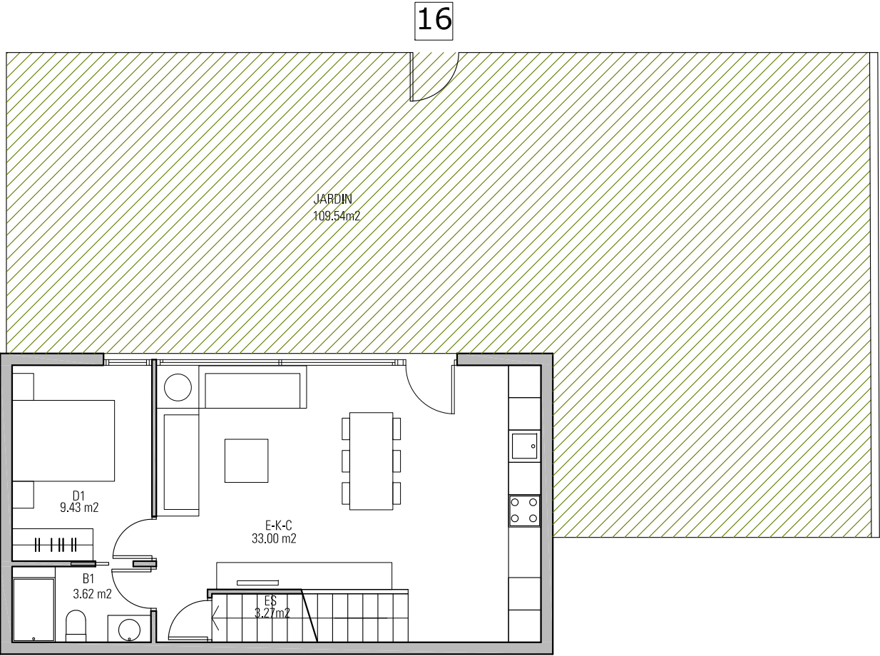
OPCION A_PLANTA BAJA
