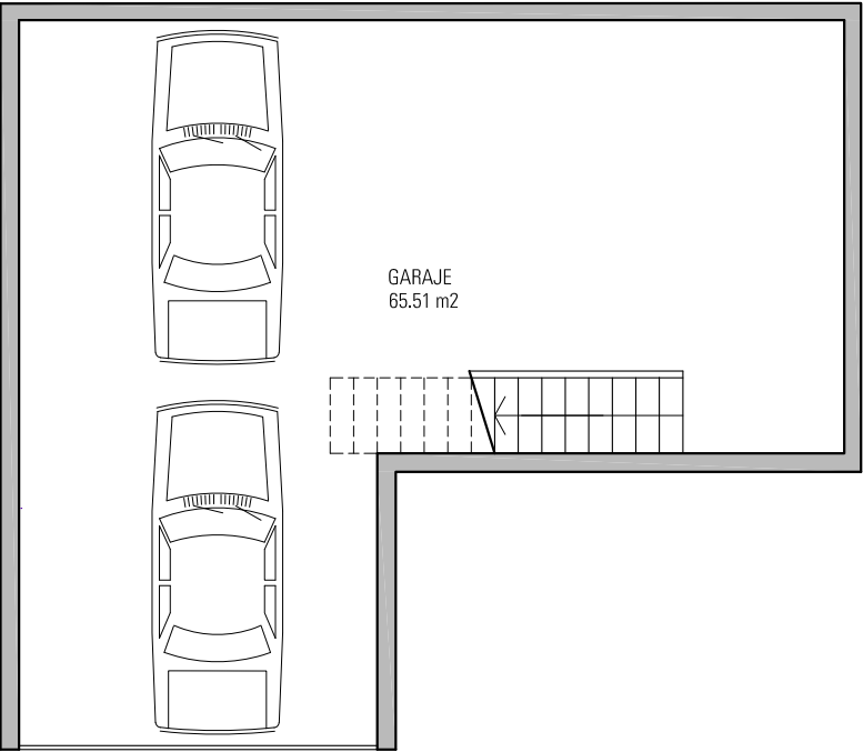
PLANTA SOTANO
