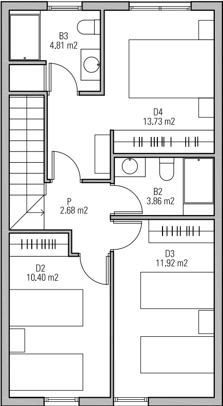
OPCION B_PLANTA PRIMERA
