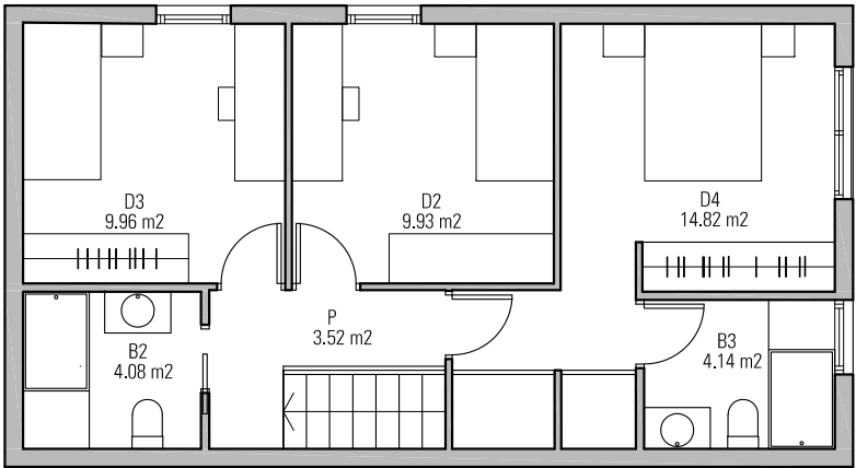
OPCION B_PLANTA PRIMERA
