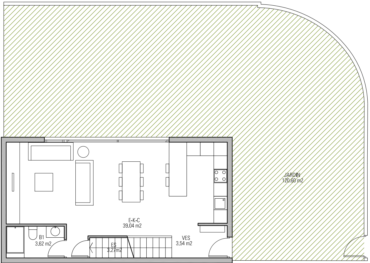
OPCION B_PLANTA BAJA
